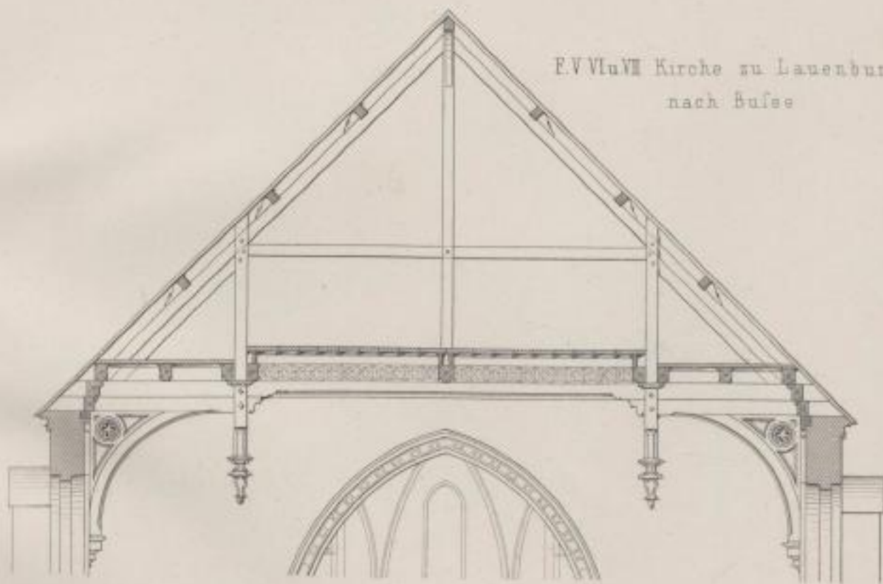
F.VI. Querschnitt
