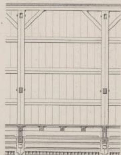
F.IV. Längenschnitt
