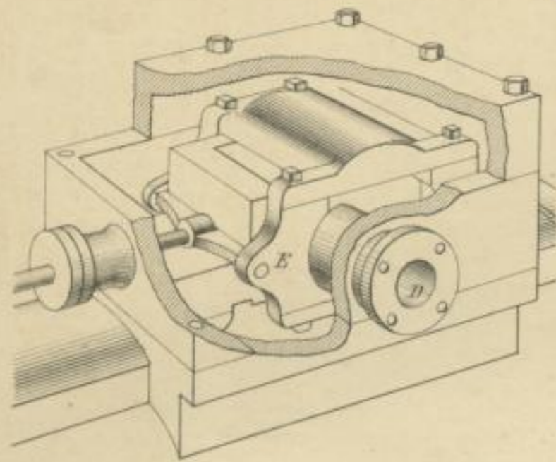
Wisner & Strong, Dampfschieber.
