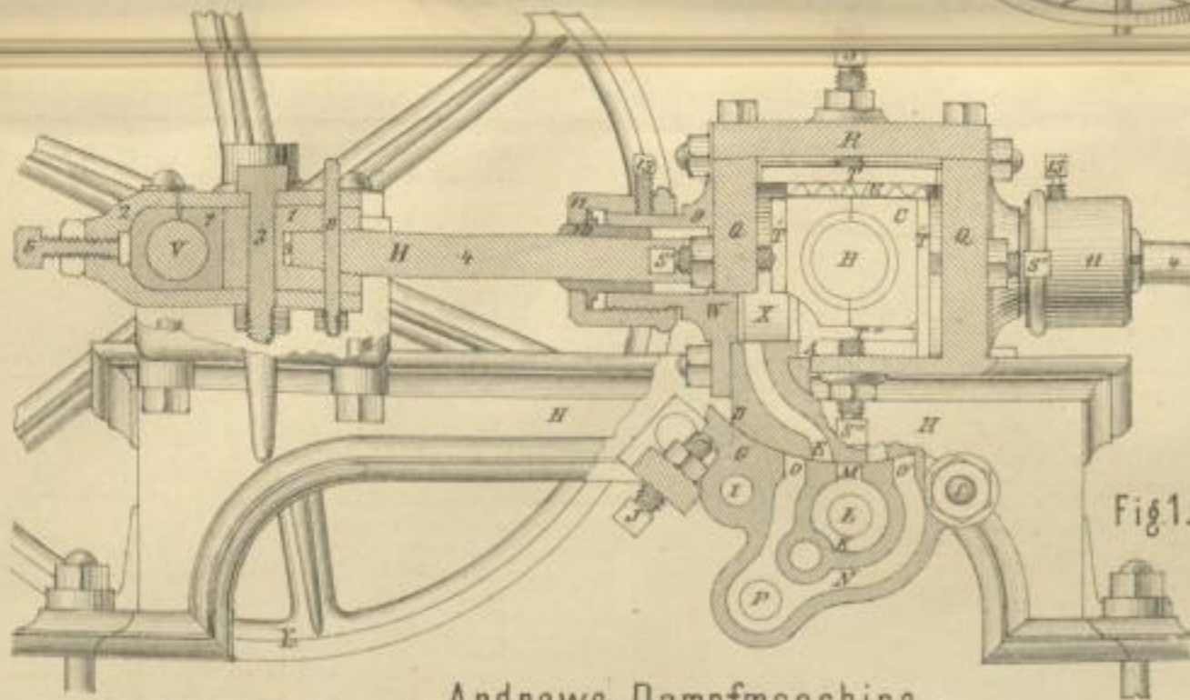
Andrews, Dampfmaschine.
