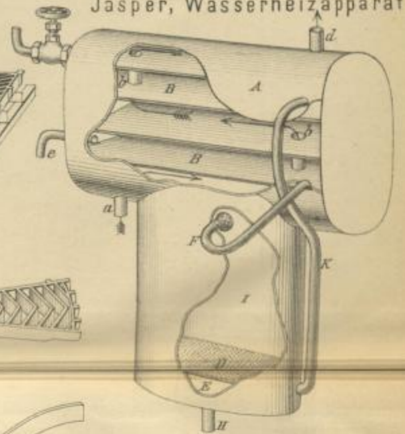
Jasper, Wasserheizapparat.
