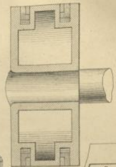
Wetherill Kolben- Packung.
