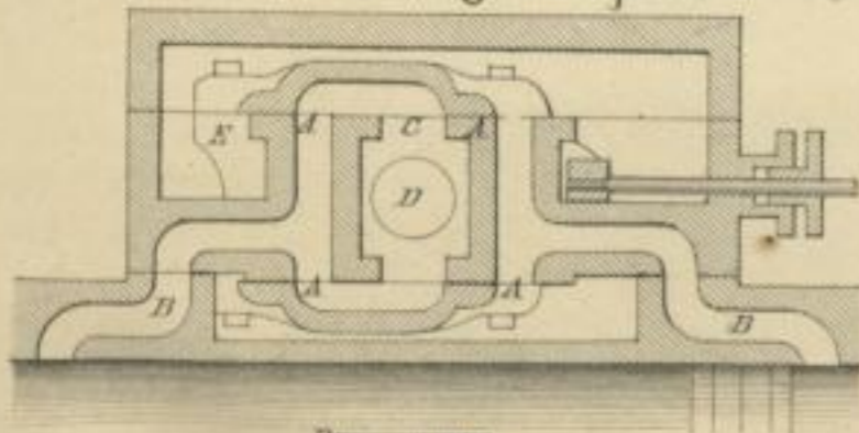
Wisner & Strong, Dampfschieber.
