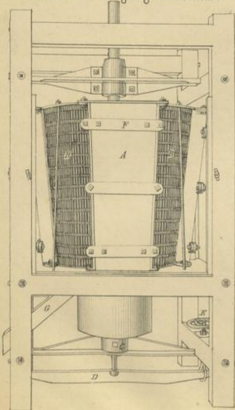
Wallace Reinigungsmaschine.
