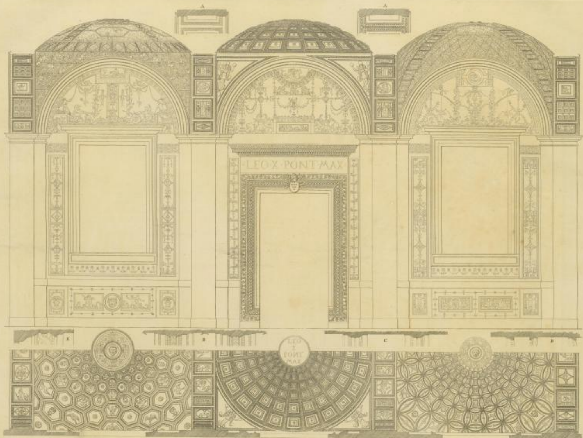
Durchschnitt von einem Theil dieser Gallerie des ersten Stockes. Coupe d'une partie de la Gallerie du premier Etage.
