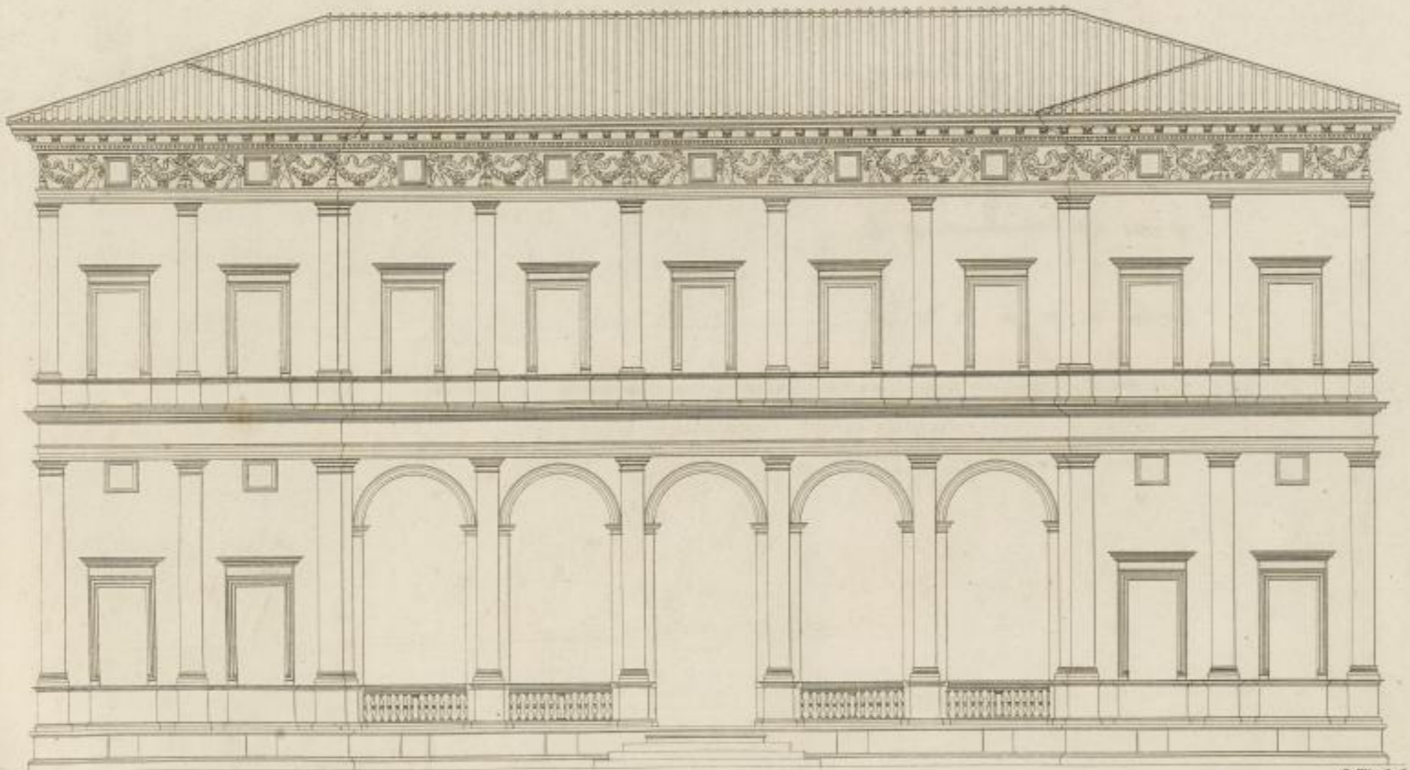
Vorder und Seiten Aufsicht vom Pallast der Farnesina. & Façade principale et laterale du Palais de la Farnesina. via della Ingara
