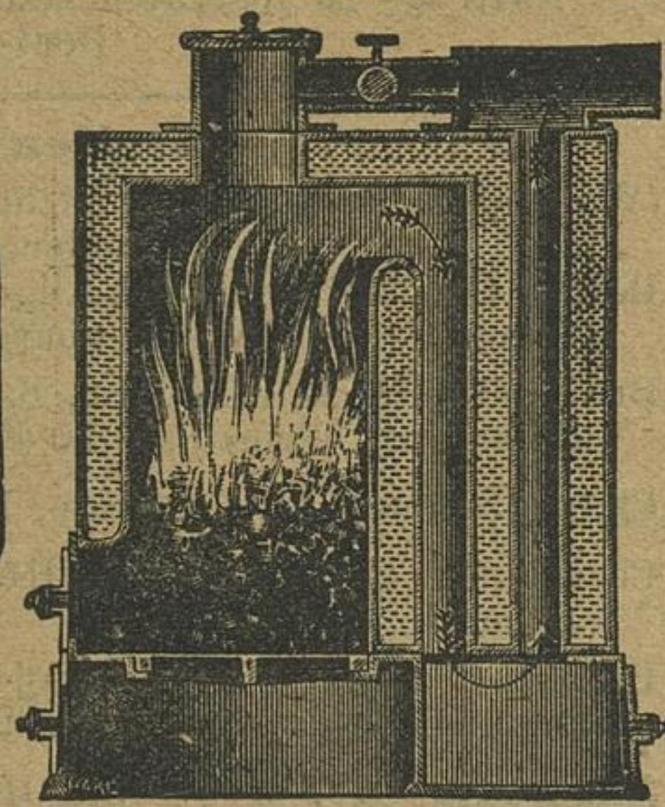
Freistehender Röhrenkessel
