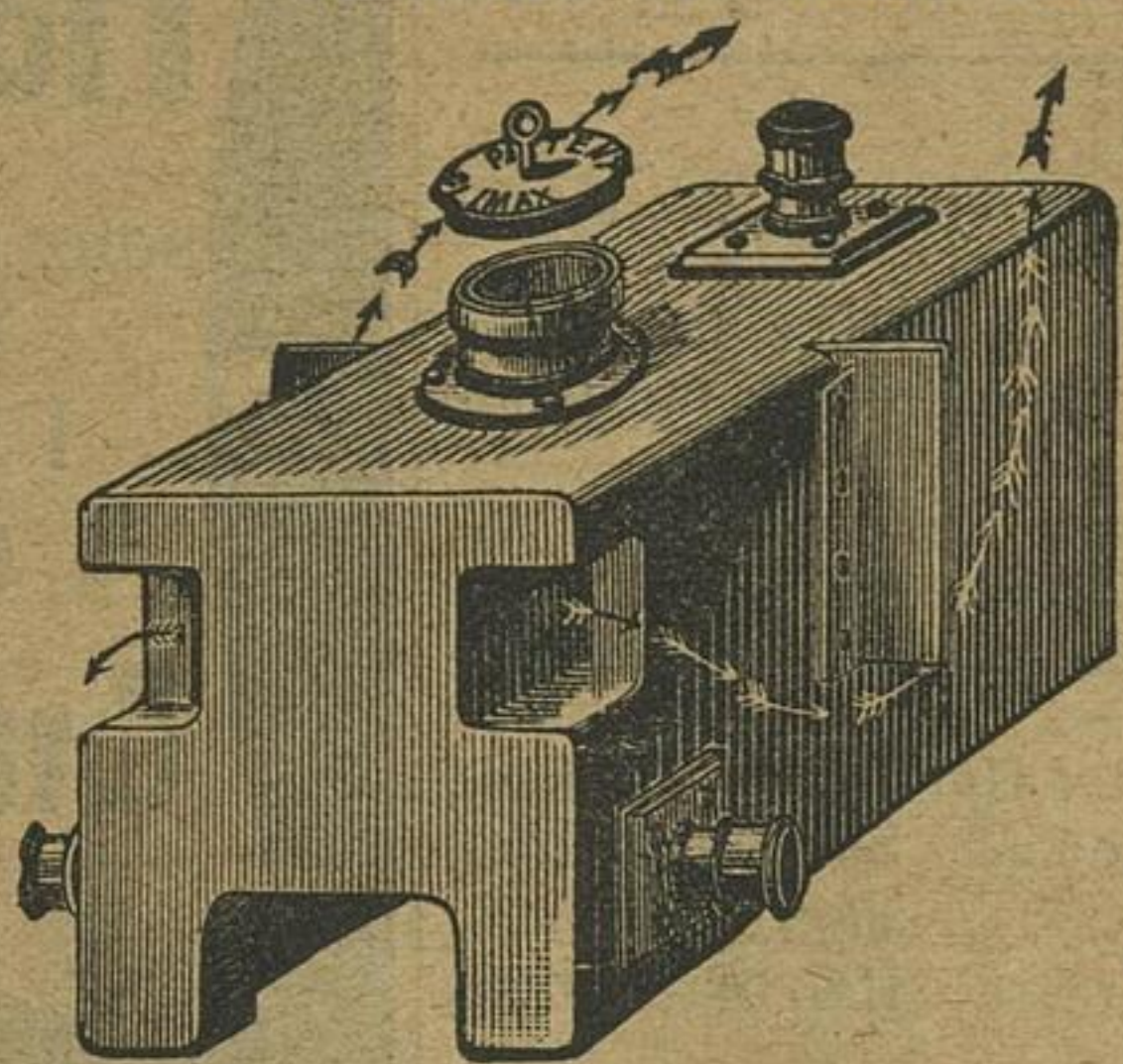
Patent-Climax-Kessel
