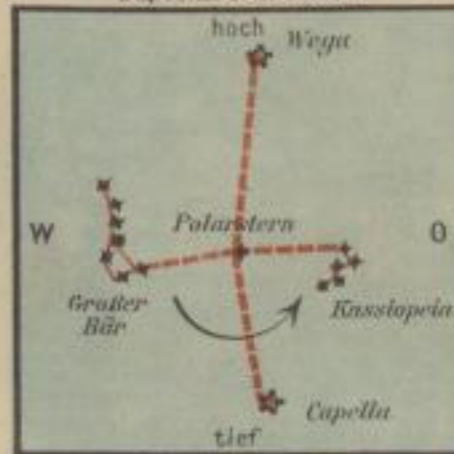
Stellung des Sternkreuzes an Septemberabenden
