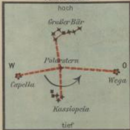
Stellung des Sternkreuzes an Juniabenden
