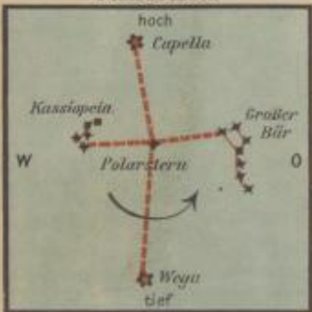
Stellung des Sternkreuzes an Märzabenden
