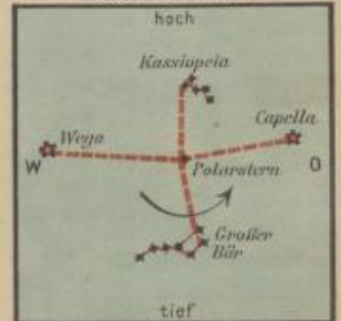
Stellung des Sternkreuzes an Dezemberabenden
