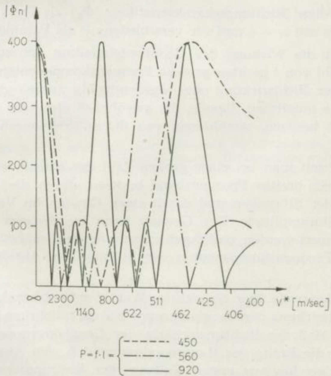
Bilder 7a und 7b. Richtcharakteristiken für Gruppen mit vier Geophonen. Umgezeichnet nach VOJUCKIJ [23]
