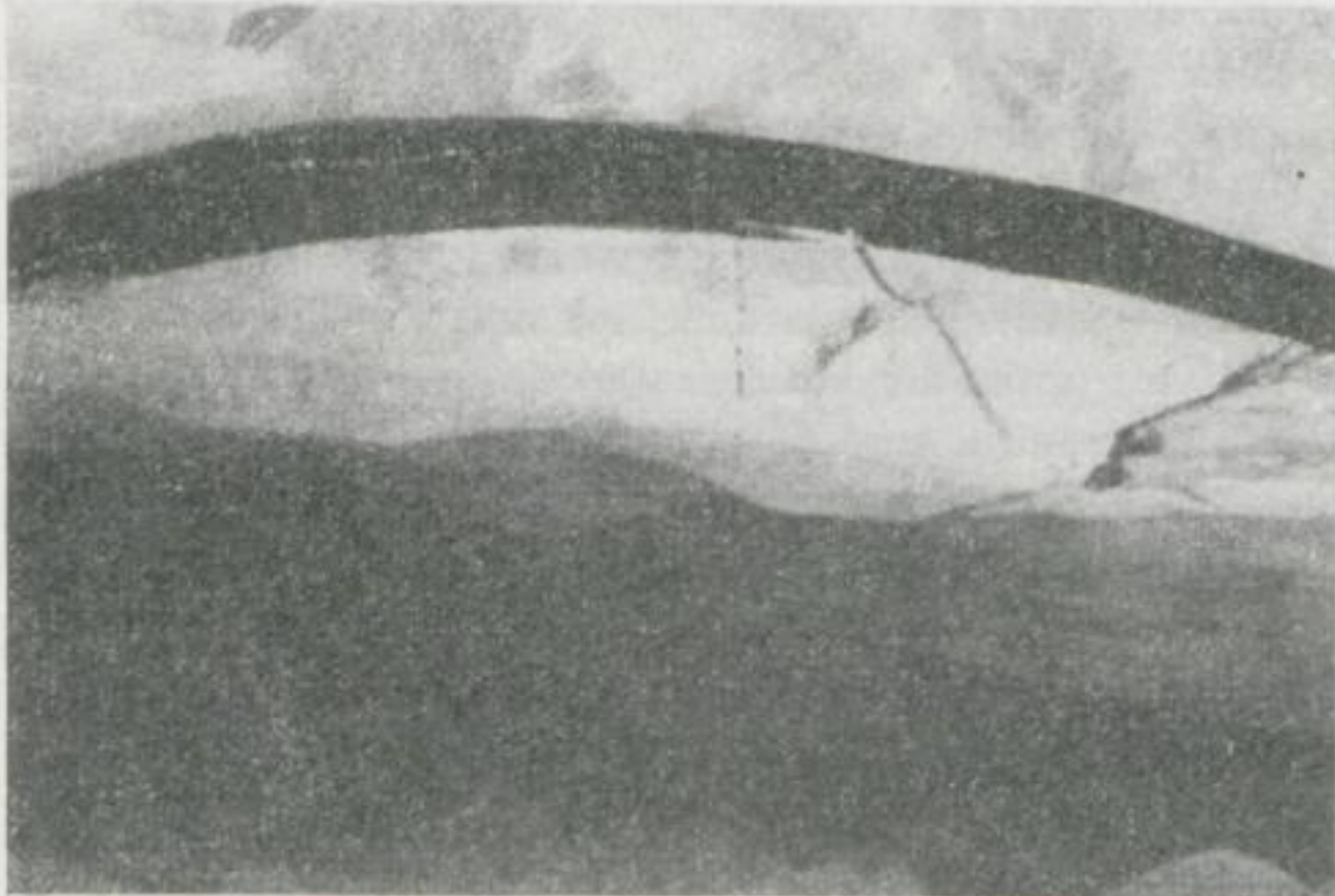
Bild 48 Gewölberiß auf Kali- werk „Friedenshall“, Bernburg
