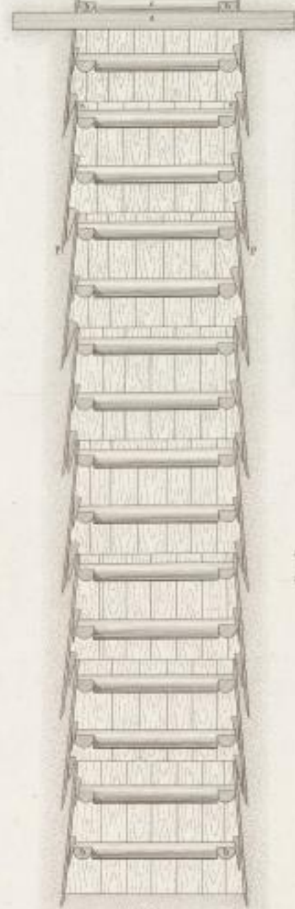
Fig. 7. Coupe verticale suivant CD des fig. 1. & 2. II°
