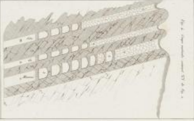
Fig. 7 Coupe verticale suivant C D de Fig. 1
