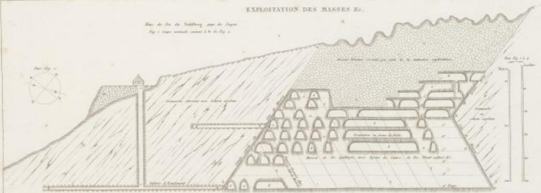
Fig. 3 Plan par un coupe A B de Fig. 1
