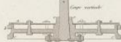
Fig. 2. Détails de l'arbre - Moteur
