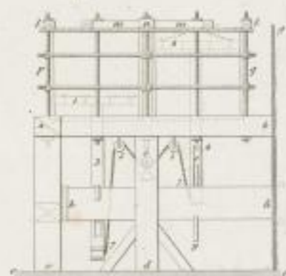
Fig. 5. Plan supérieur.
