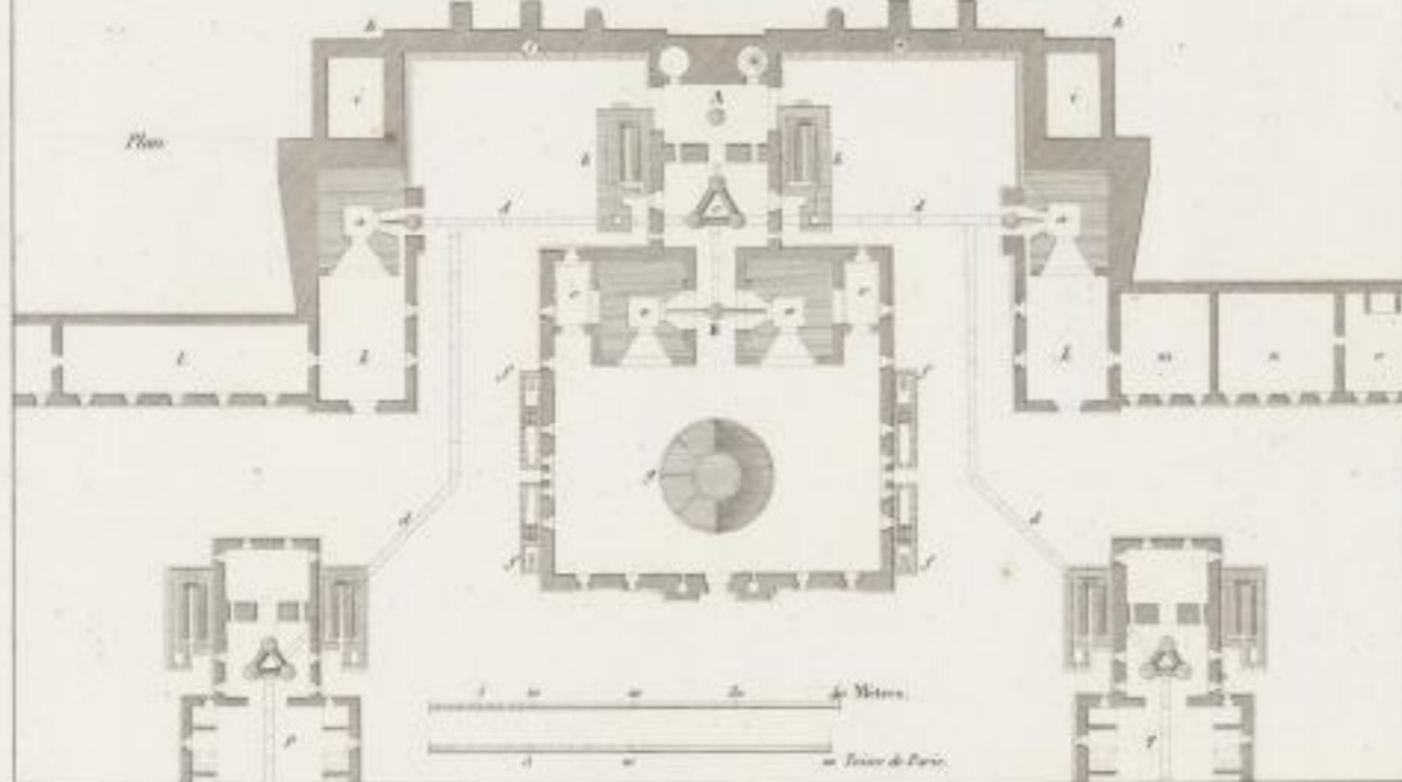
Fig. 3. Usine à fer dite le Grand , Dép. de Seine et Loire, Foyes. Fig. 8. et 9.
