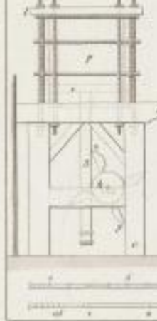
Fig. 6. Elevation latérale.
