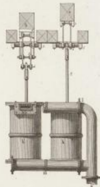
Fig. 3. Elevation suivant CD de Fig. 1.
