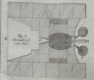
Fig. 26 Durchschnitt nach RS der Fig. 25.
