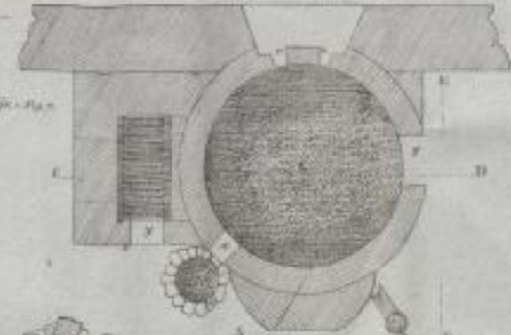
Fig. 7 Grundriss nach Fig. 5.
