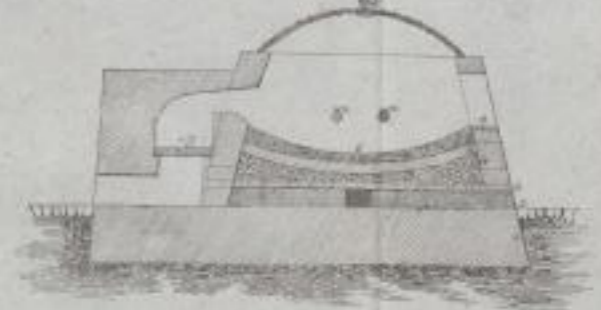
Fig. 6 Durchschnitt nach CD der Fig. 5.
