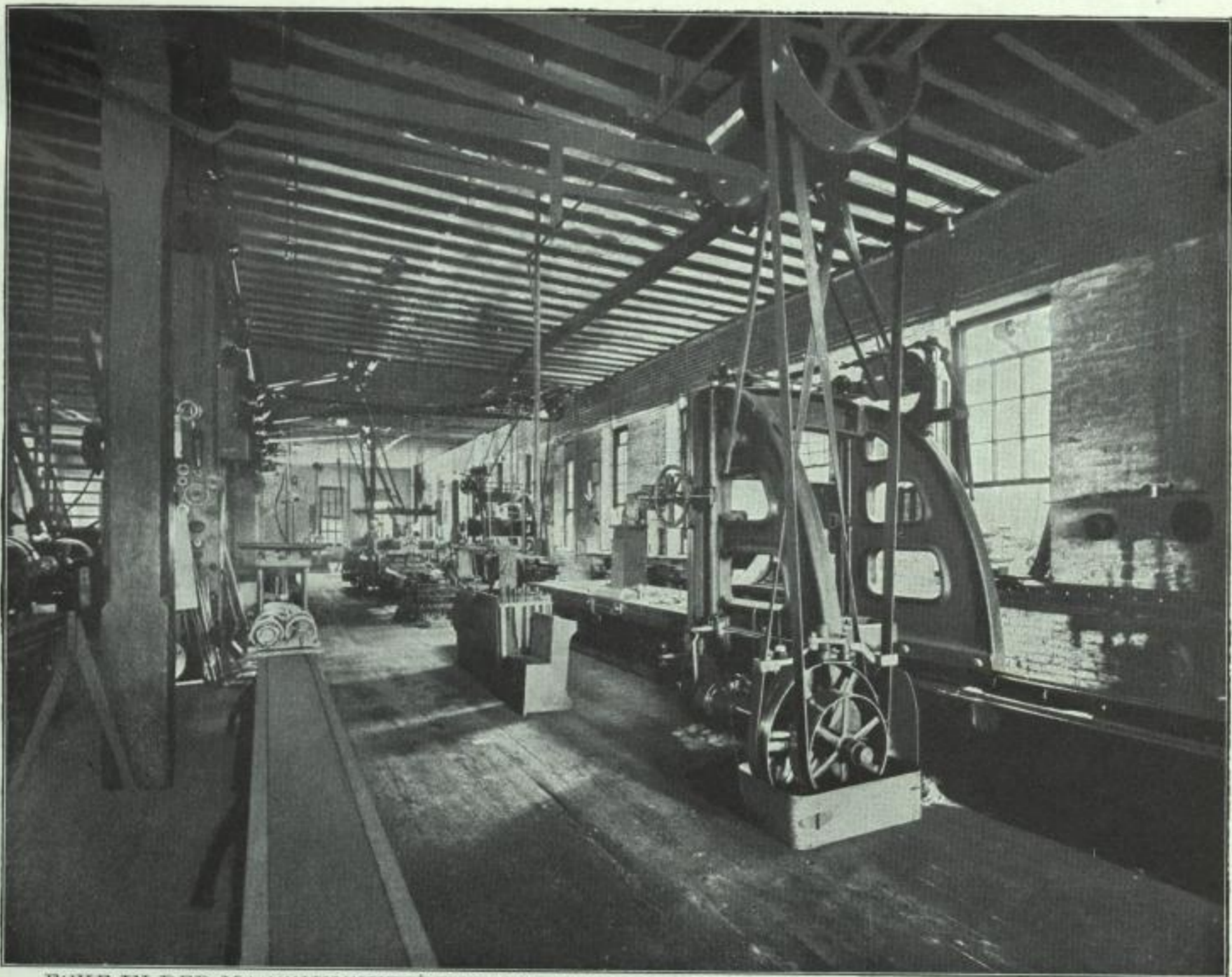
ECKE IN DER MASCHINENWERKSTATT—MEHRERE METALL-HOBELMASCHINEN ZEIGEND.
