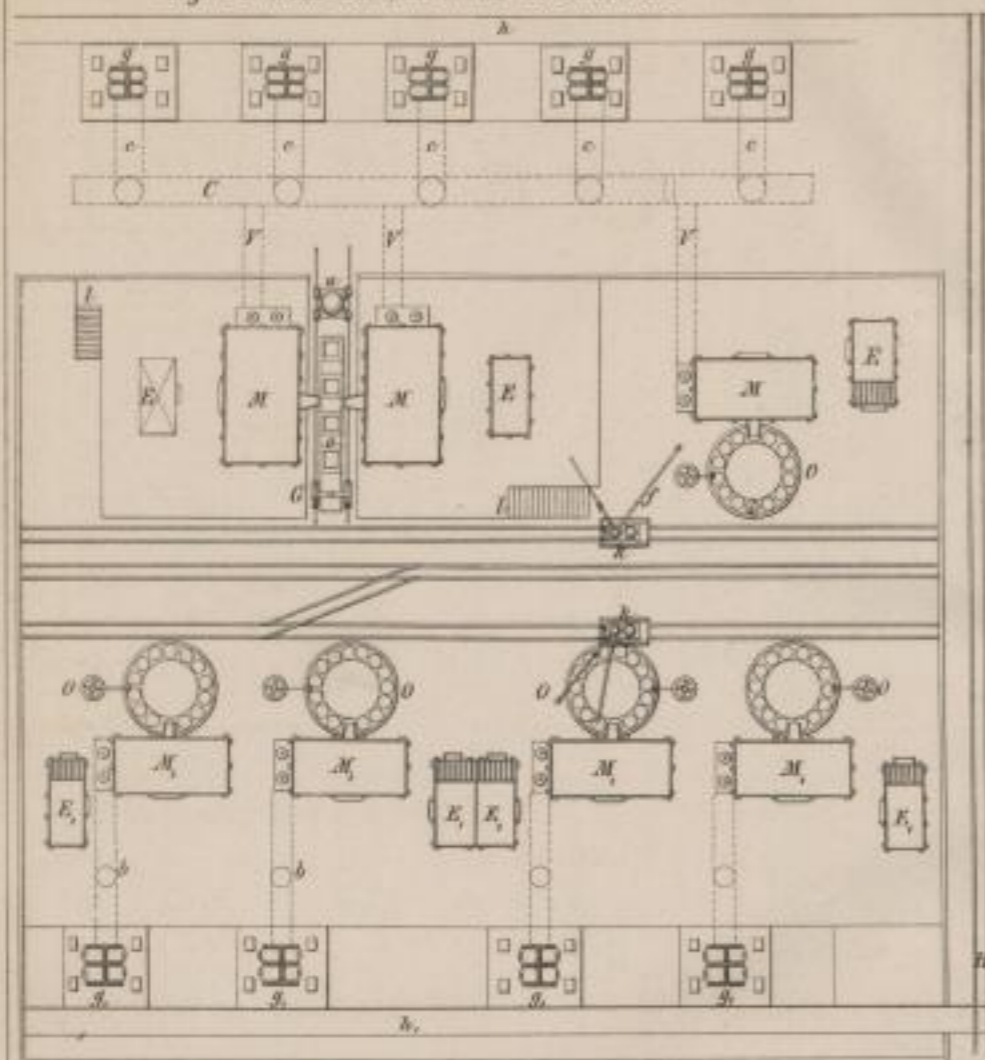
Fig. 1. Martin-Siemens-Hütte in Terrenoire.
