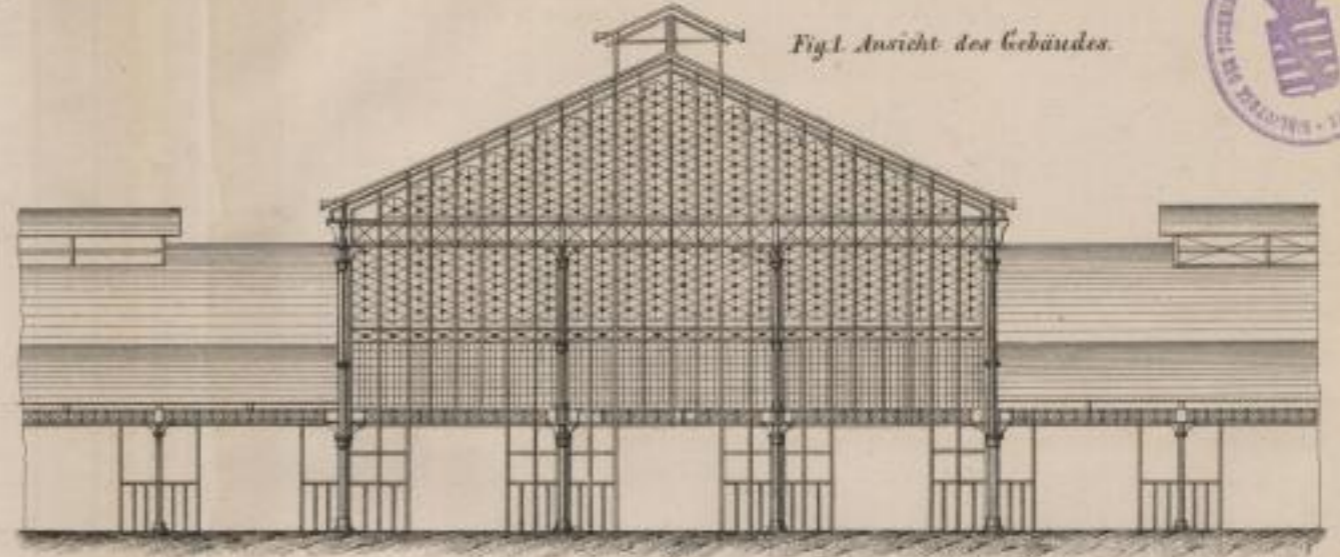
Die Anlage des 80-Tonnen-Hammers in Creusot. (Fig. 1-3.)
