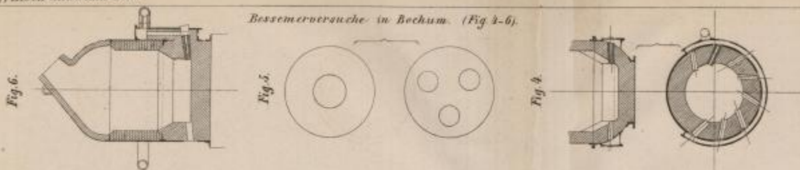
Fig. 2. Vorder-Ansicht.
