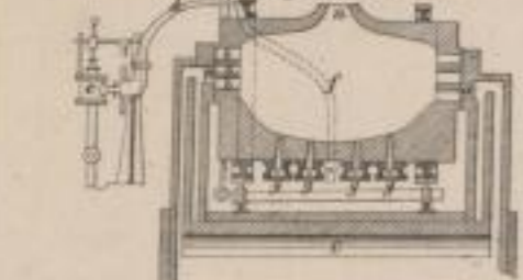
Fig. 11. Querschnitt.
