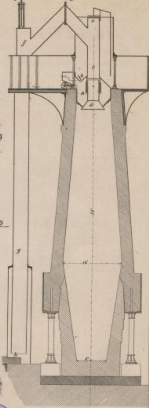
Hohofen in Vordernberg Fig. 3.
