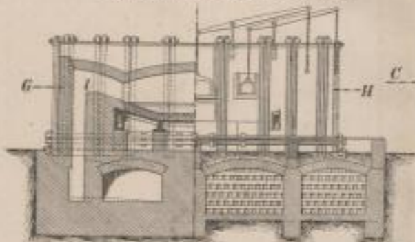
Fig. 6. Schnitt A B. Vordere Ansicht.
