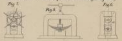
Fabrikation von Stahlfedern in Forming (Fig. 5-8)
