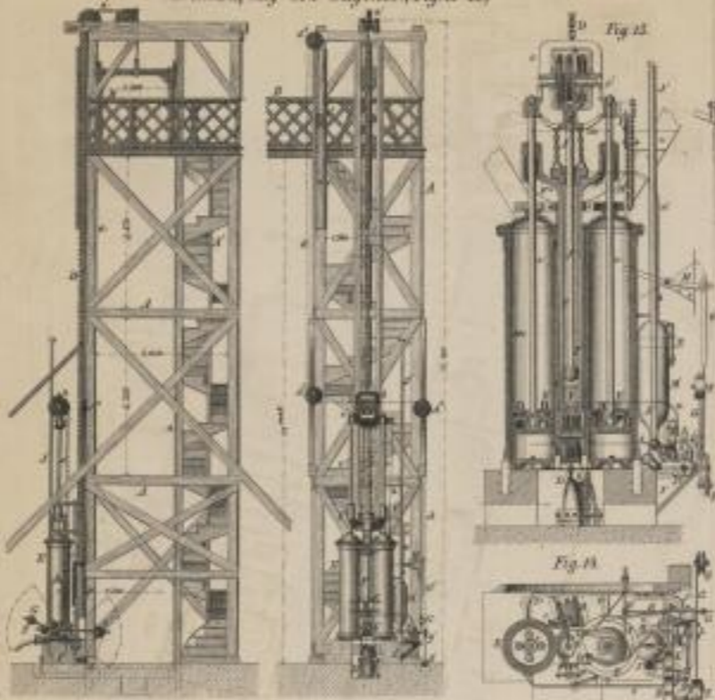
Gichtaufzug von Guyenet (Fig. 11-15)
