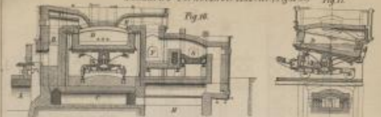
Hofenanlage in St. Louis.
