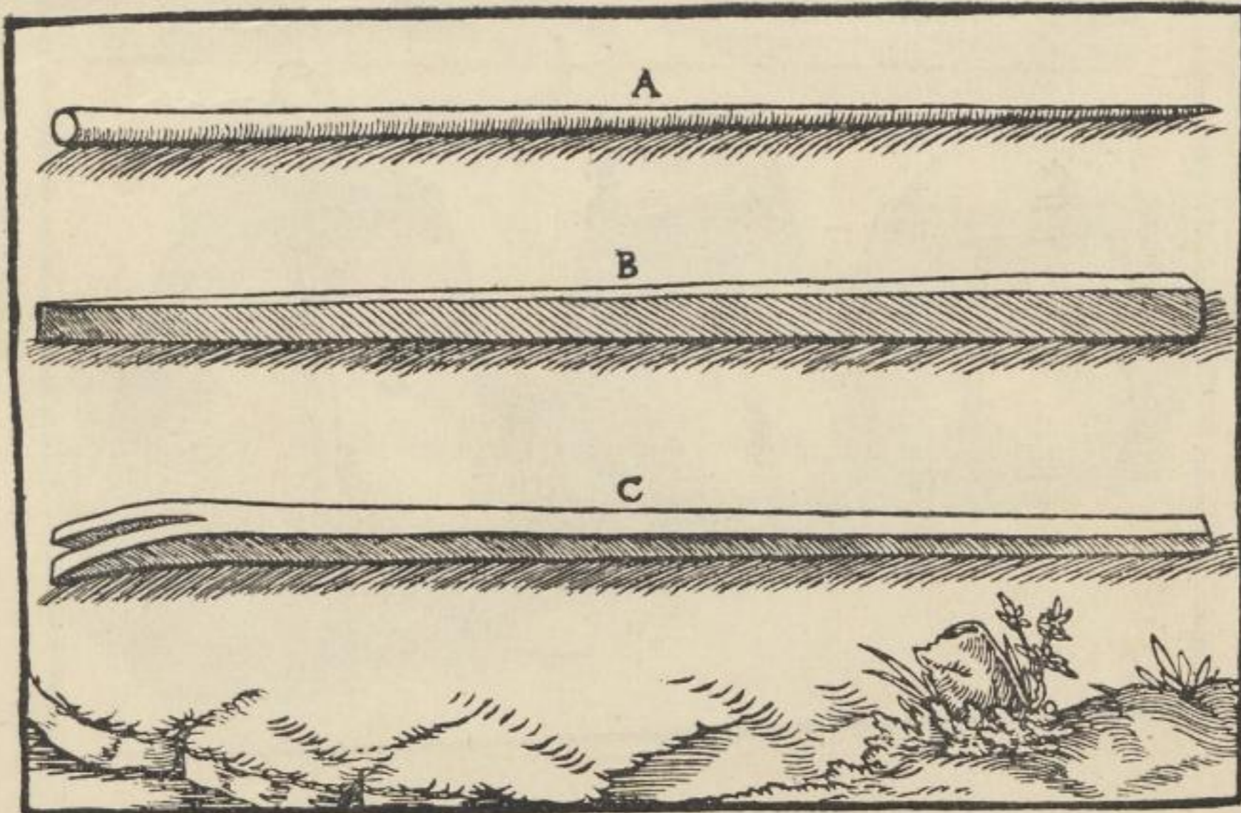
Bild 4. Das Eisen zum Durchschlagen A. Das Brecheisen B. Die Brechstange C.
