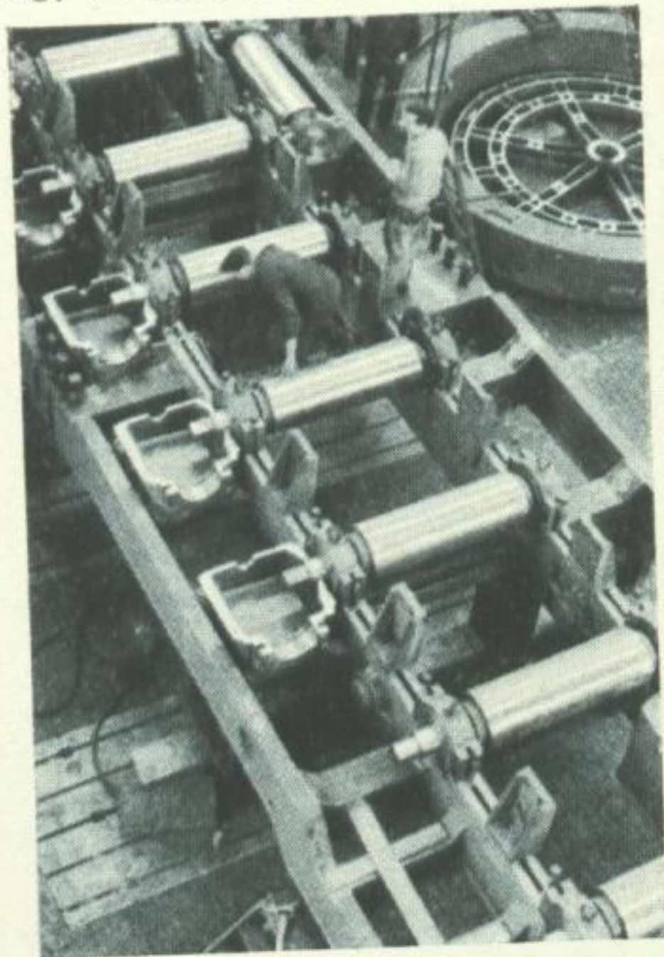
Egy hengerso szerelése
