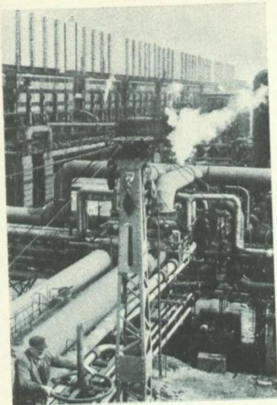
A lauchhammeri barnaszén- kokszoló
