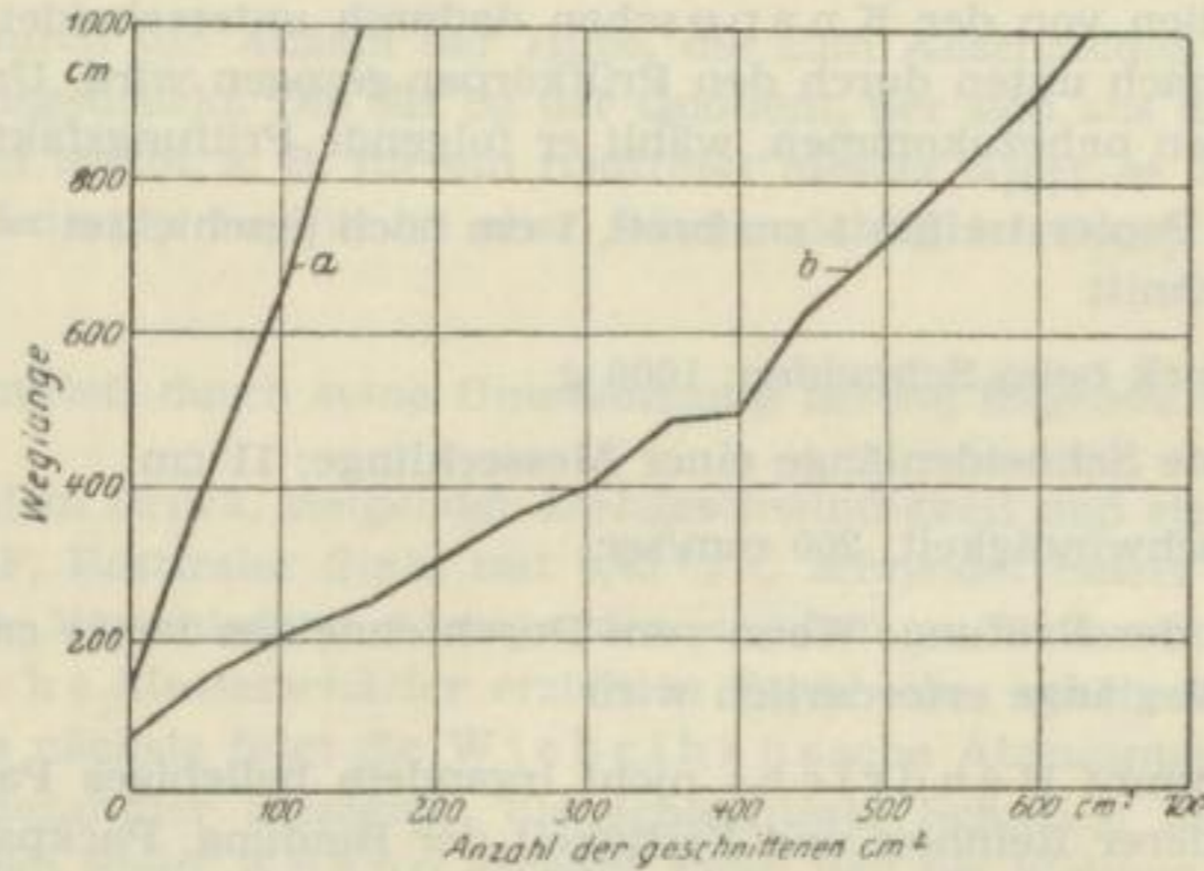
Bild 4. Arbeitsleistung in Abhängigkeit von der Weglänge der Schneide (nach F. Hendrichs)
