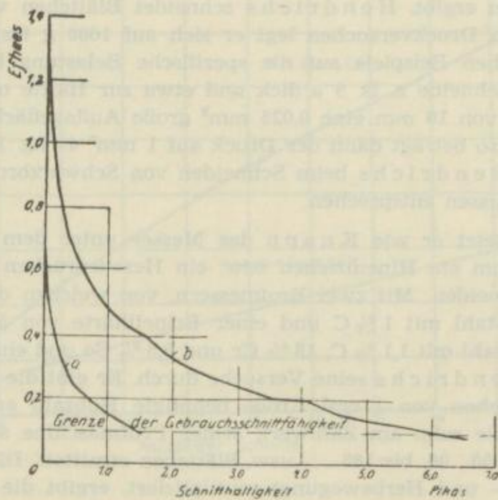
Bild 5. SF (Efhaës) und SH (Pikas) der Messerklingen (nach F. Hendrichs)
