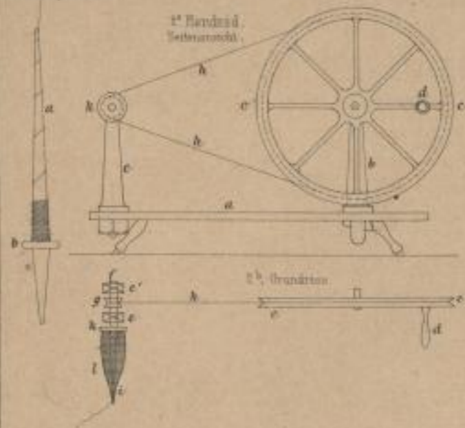
1. Handspindel (H.)
