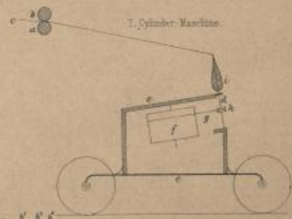
5. Mule-Maschine (Crompton 1779)
