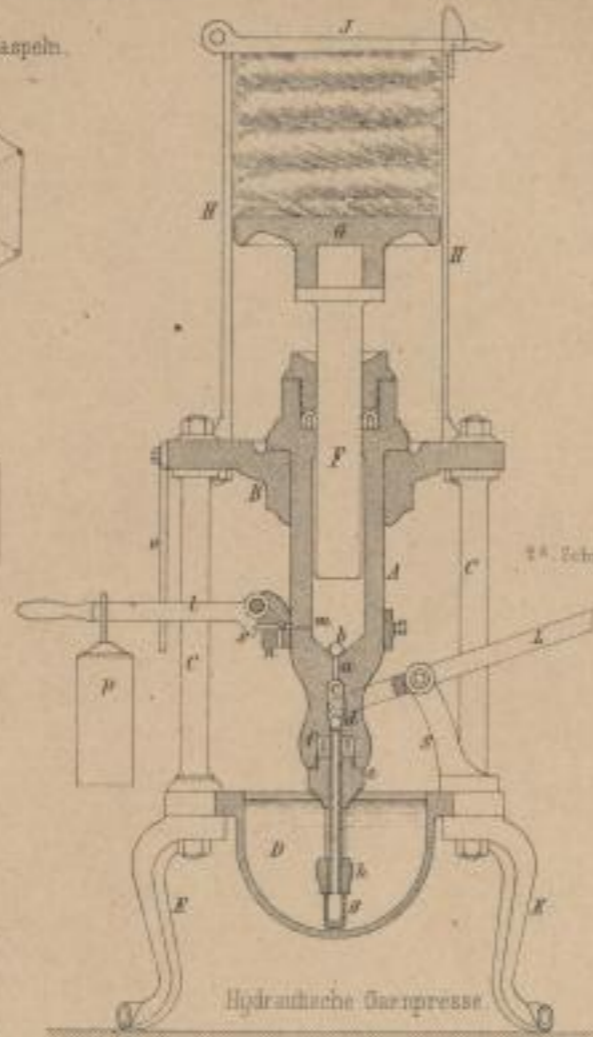
3a Vorderansicht
