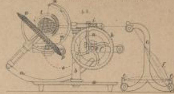
4a Vorderansicht
