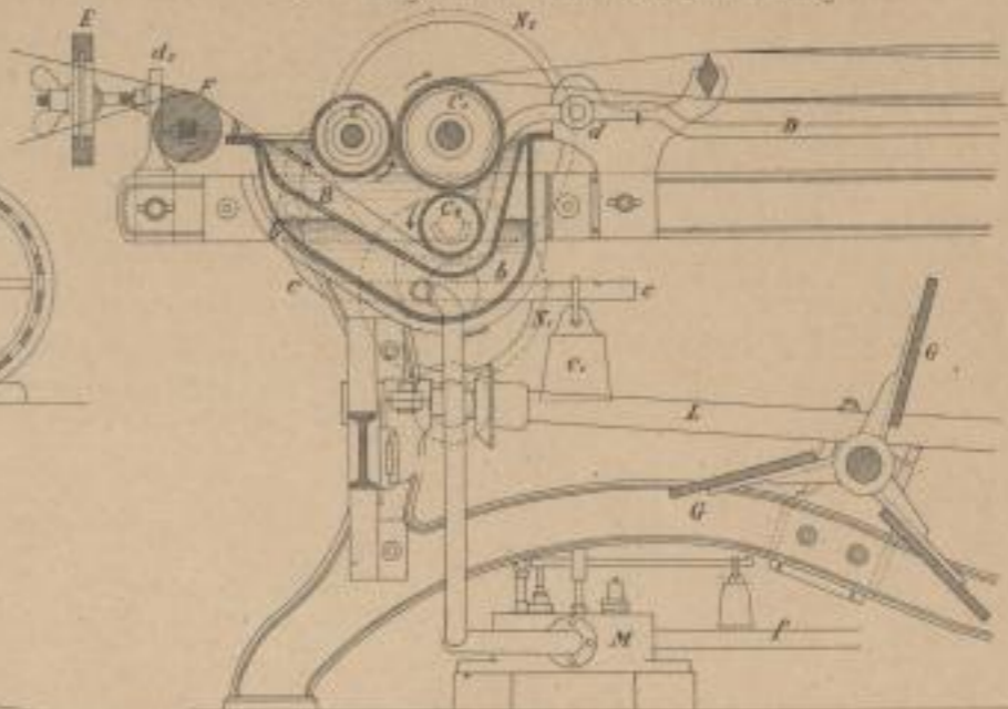
3 b. Längenschnitt durch den Schlichterog
