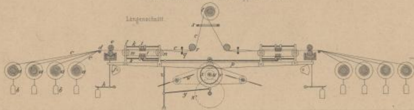
1. Schlichtmaschine mit Bürstenapparat. 3. 150.
