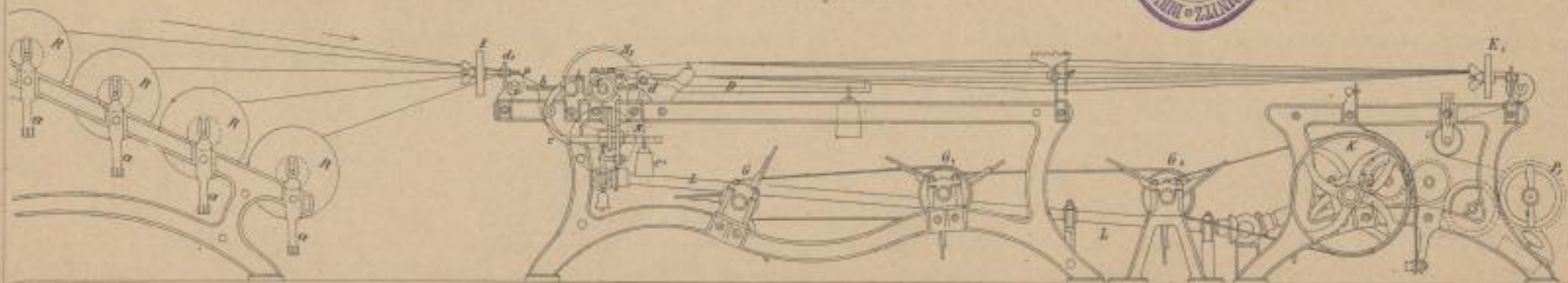
3. Schlichtmaschine mit Luftzug-Trockenapparat v. Fassin.
