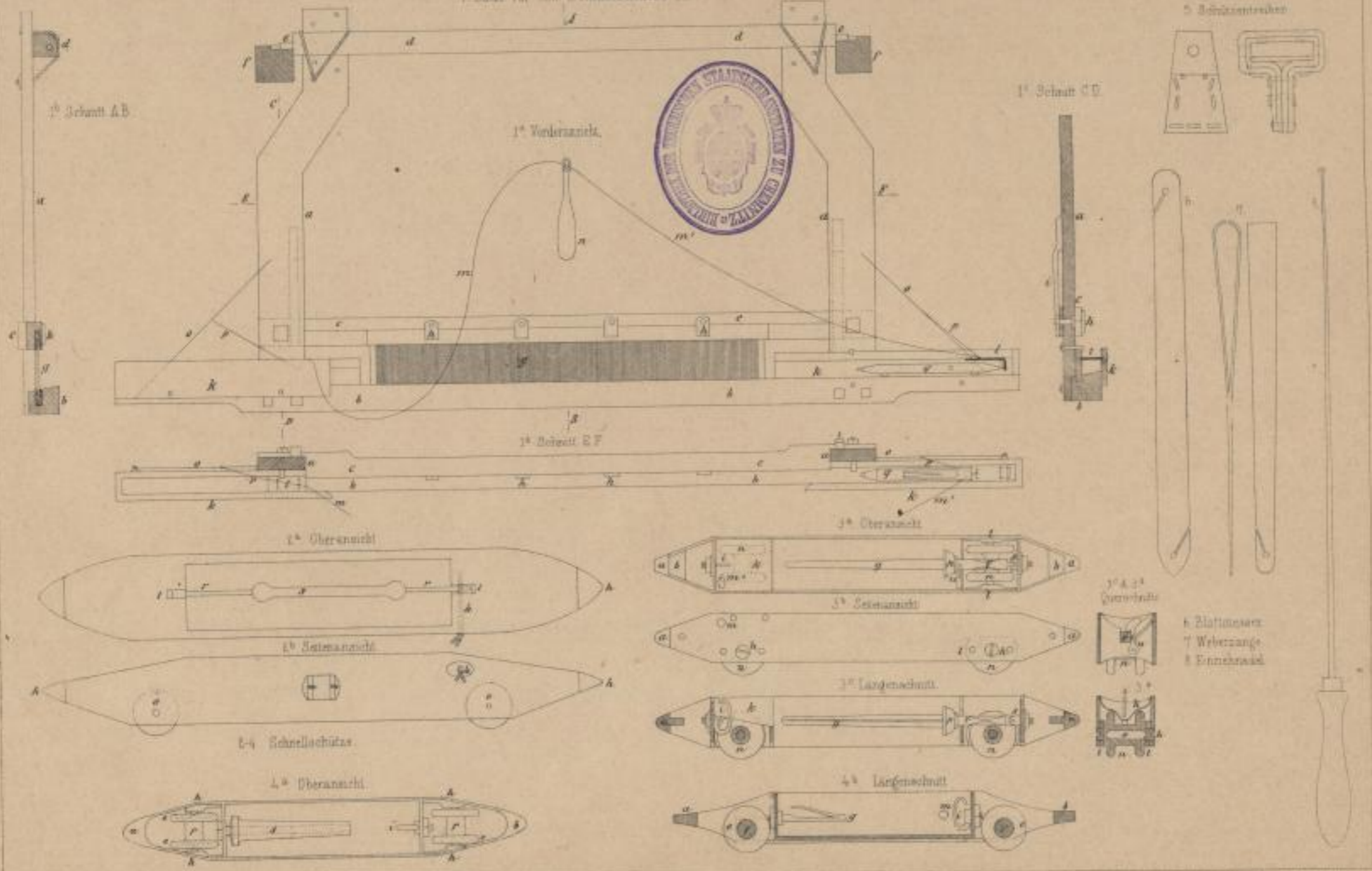
1. Lade für eine Schnellschütze (No. 1)
