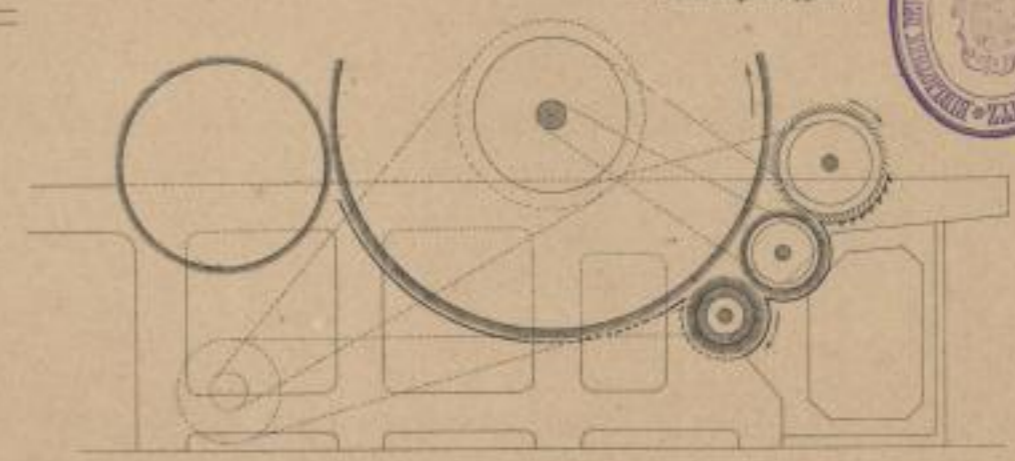
5. Trommelputzapparat
