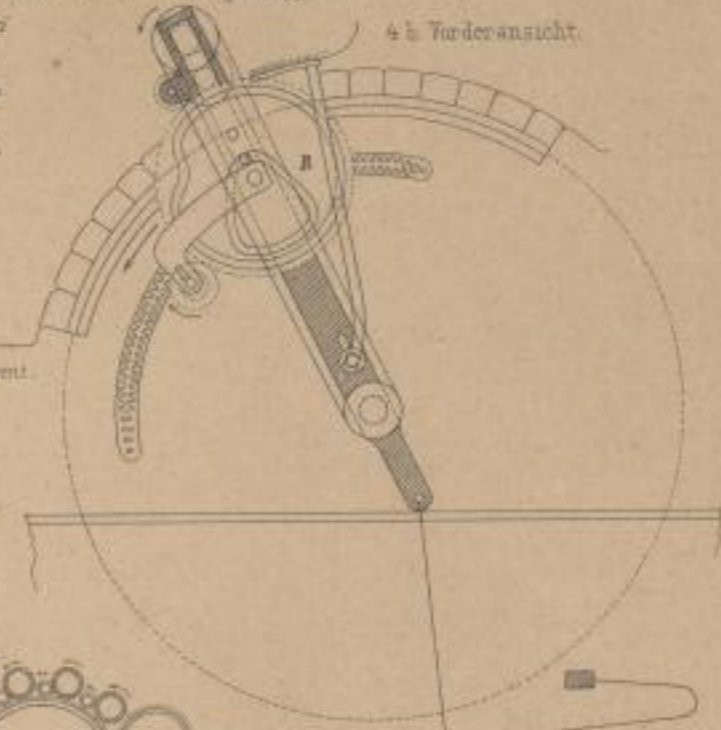
4. Weilmann's-Deckelputzapparat
