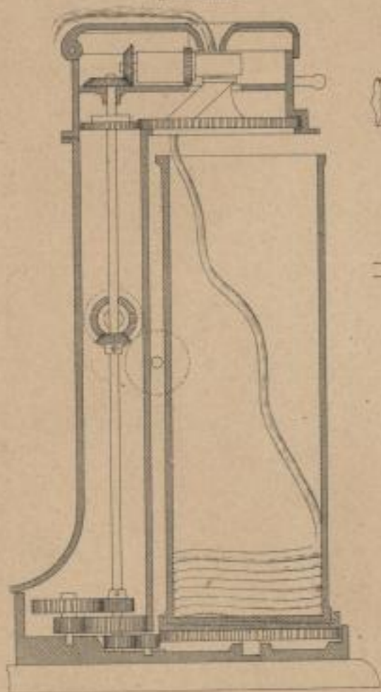
1b Lage der Windungen im Topf
