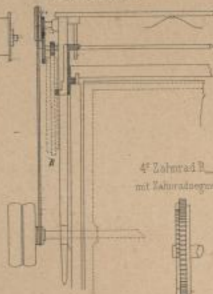
4a Seitenansicht
