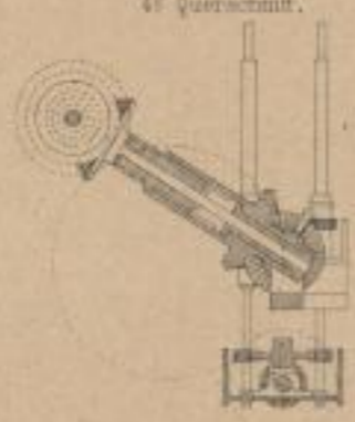
4 b Querschnitt.
