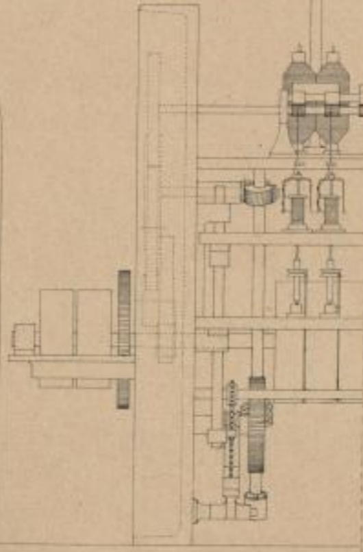
7 Längen Ansicht
