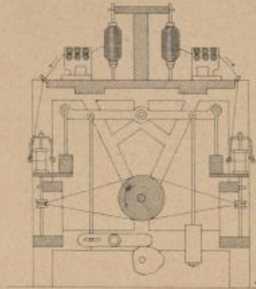
5 Watermaschine Querschnitt
