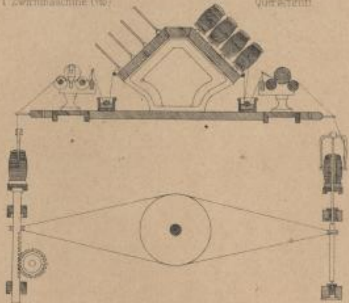
3. Querschnitt
