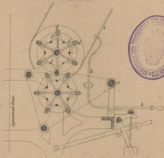
3. Querschnitt
