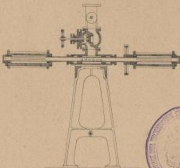
2 a Seitenansicht
