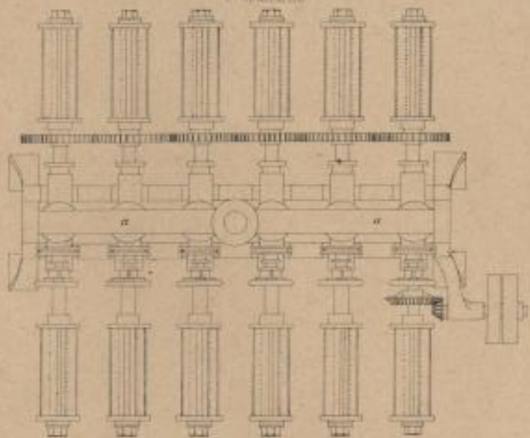
2. Gärtnerschmaschine
