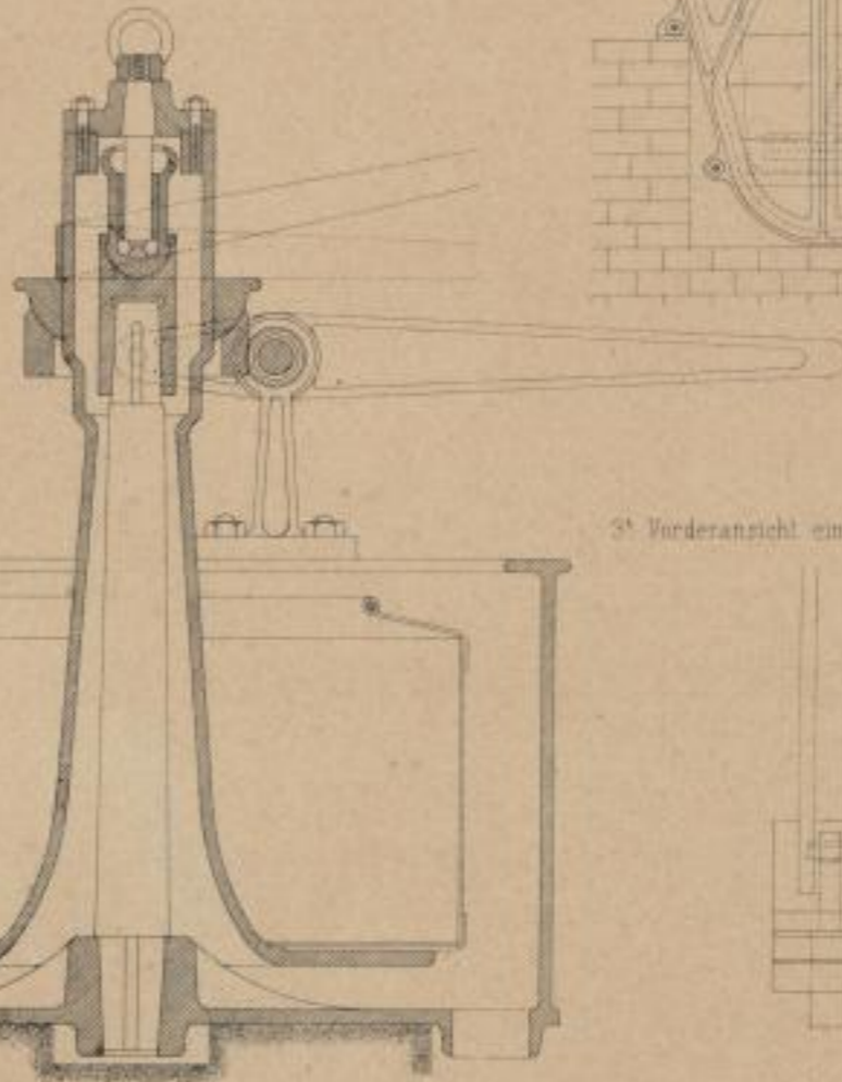
4 Centrifuge Vertikalschnitt
