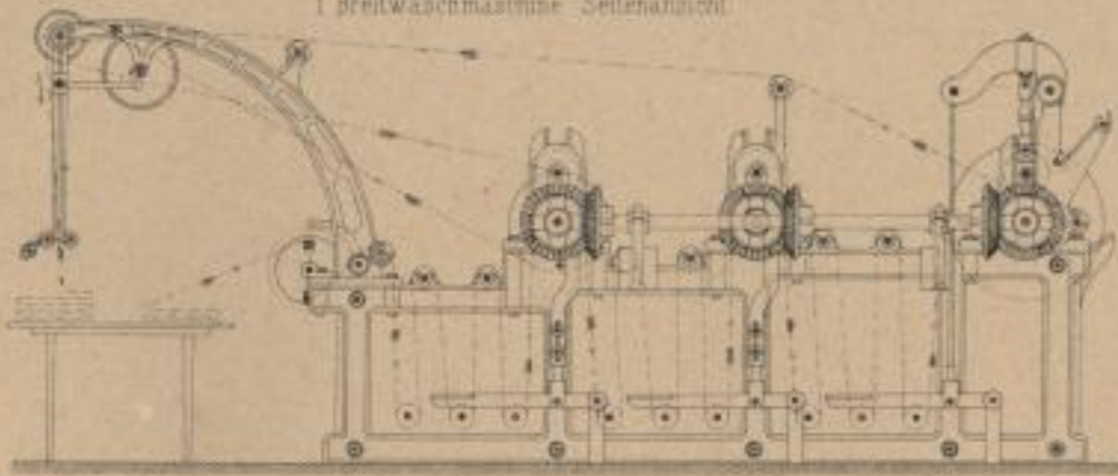
1 Breitwaschmaschine Seitenansicht
