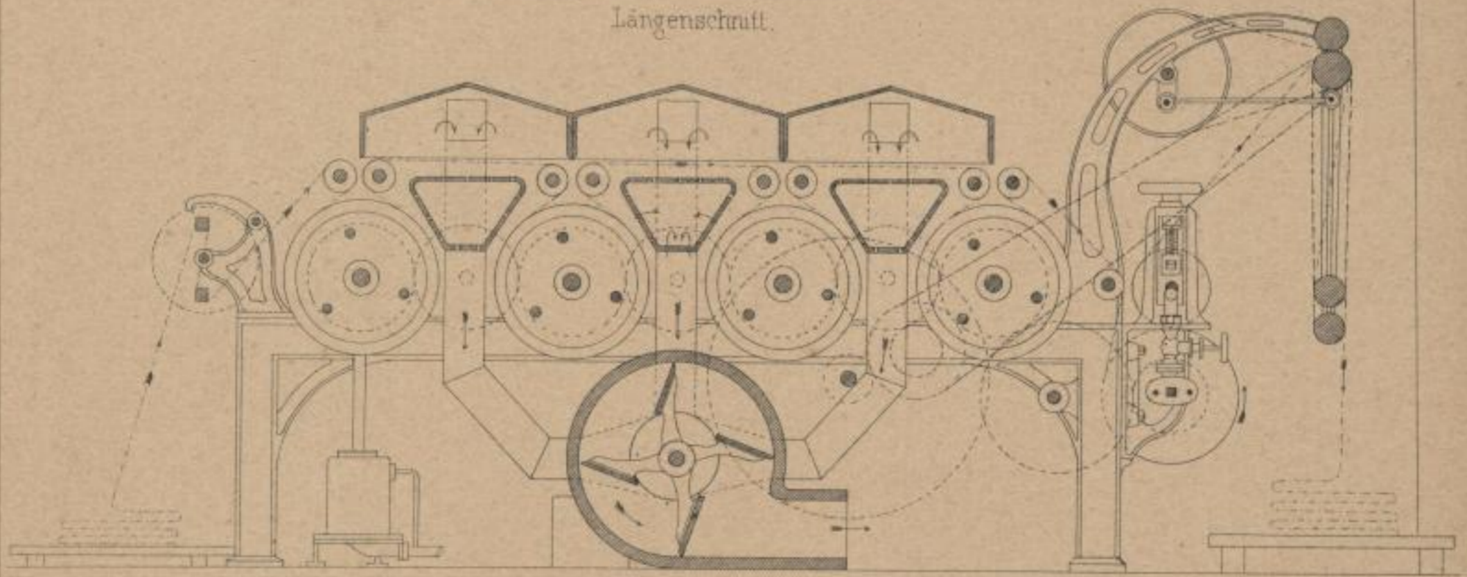
3. Trockenmaschine mit 4 Trockencylinder und Ventilation für gestärkte und ungestärkte Gewebe
