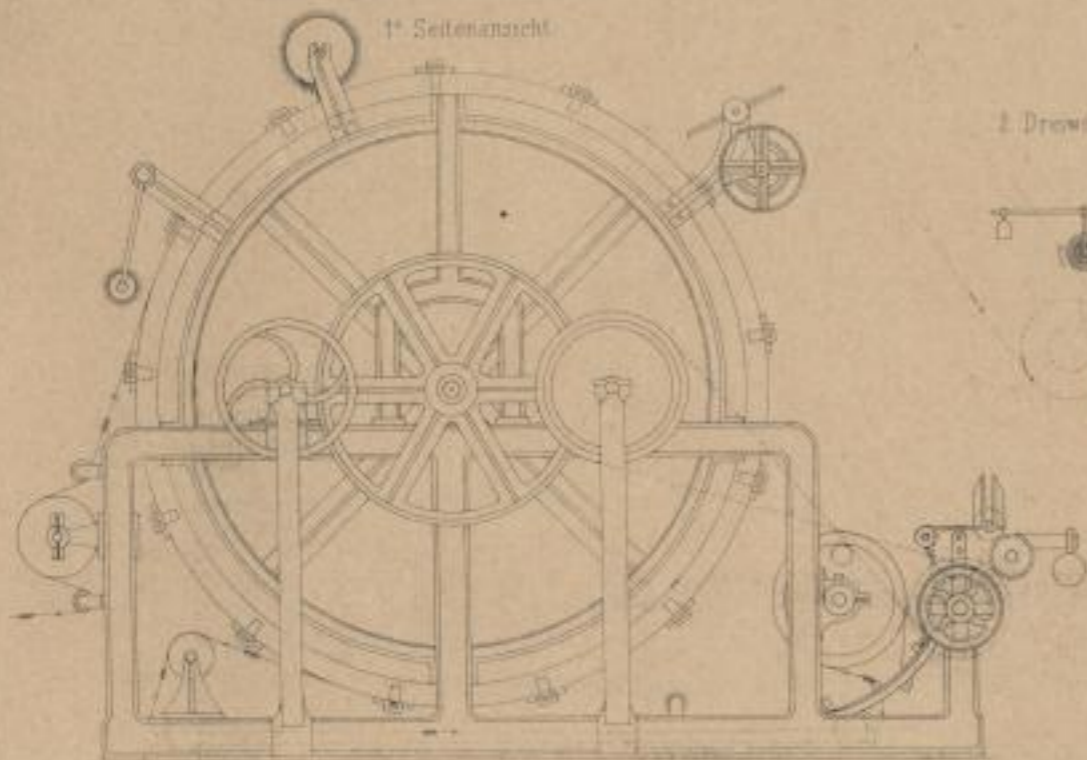
1 Cylinder-Spann- u. Trockenmaschine
