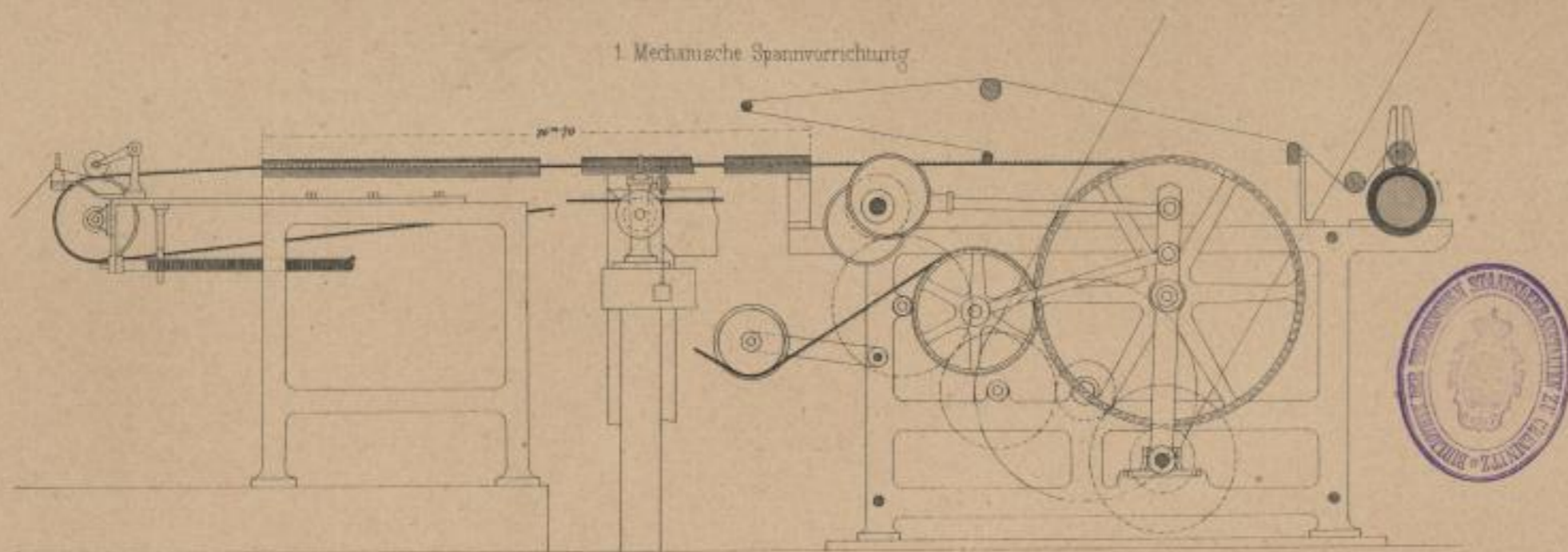
2. Doublet Maschine mit Mess- u. Aufrollapparat
