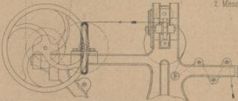
2 a Seitenansicht
