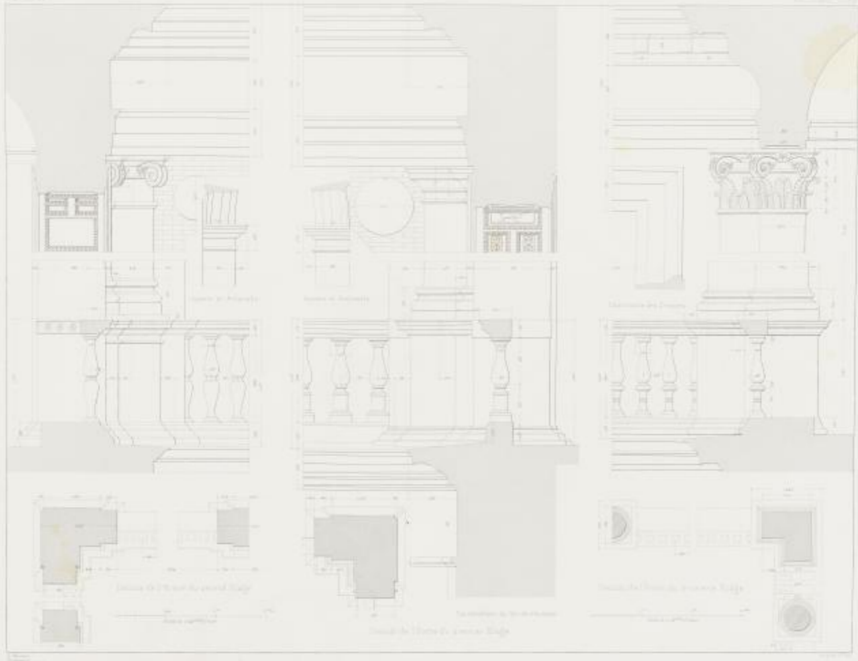
DÉTAILS ARCHITECTURAUX DE LA LOGE DE LA GAMMA DES COUPE DES LOGES
