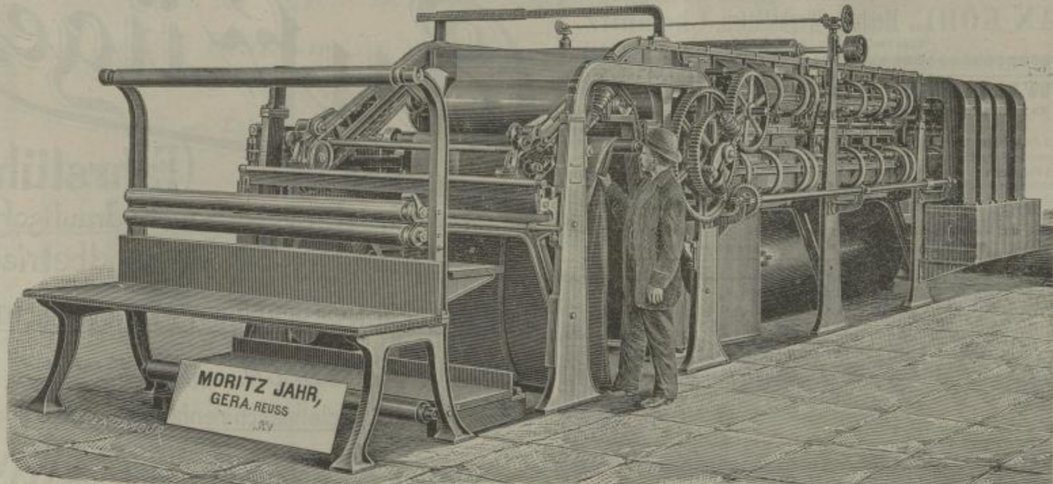
Neueste Tuchtrockenmaschine mit Lufttrocknung in Verbindung mit directer Röhrenheizung.
