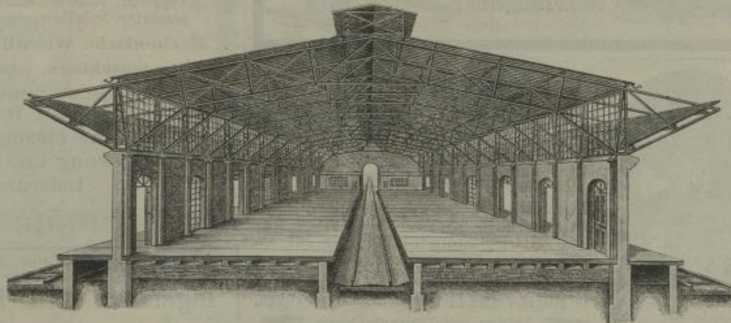
Eiserne Dachconstruction eines Güterschuppens, mit Wellblecheindeckung.
