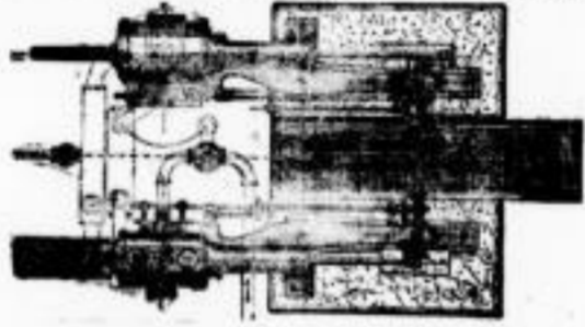
Dampfmaschinen mit Collmann-Steuerung.
