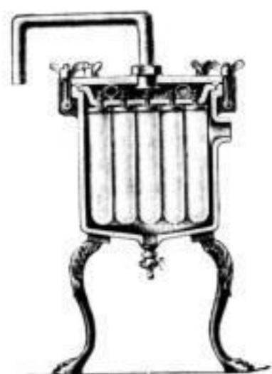
Filter-Louis mit 3 bis 50 Cylindern, überaus gute Leistung, bis 200 Liter pro Minute.
