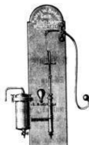
Samson-Filter besteht aus Filterkopf und Zentrifuge für Wasser, Wein u. s. w.
