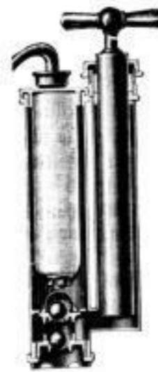
Reiner-Filter zur Filtration auf Wasser und Wein.
