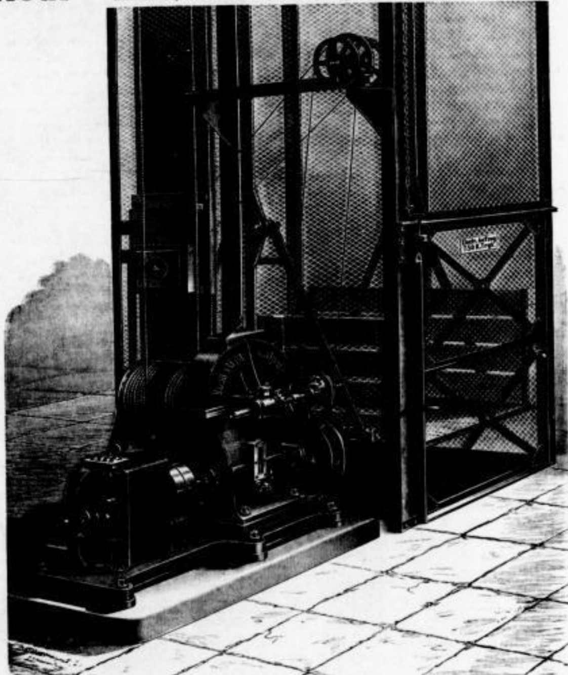
Abbildung eines der 4 electricischen Präcisions-Aufzüge im neuen Geschäftshause der Commissionbuchhandlung „K. F. Köhler“ in Leipzig.
