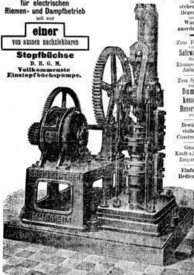
Doppeltwirkende Speise-Pumpe mit electrischem Antrieb.
