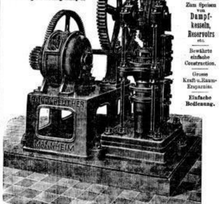
Doppeltwirkende Speise-Pumpe mit electrischem Antrieb.
