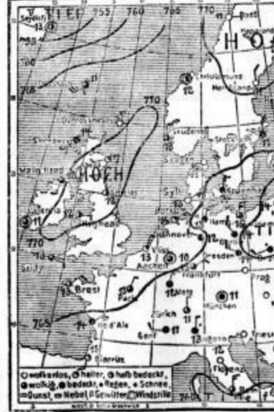
Wetterkarte vom 8. September.
