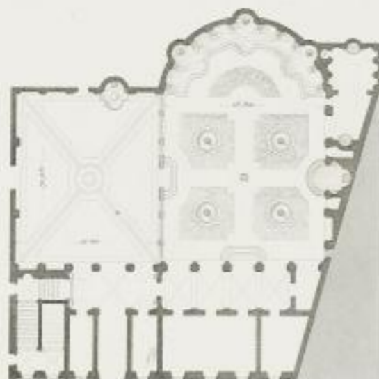
Plan de l'habitation et de la Nymphée du Collège Nucerino, n. II. 20.
