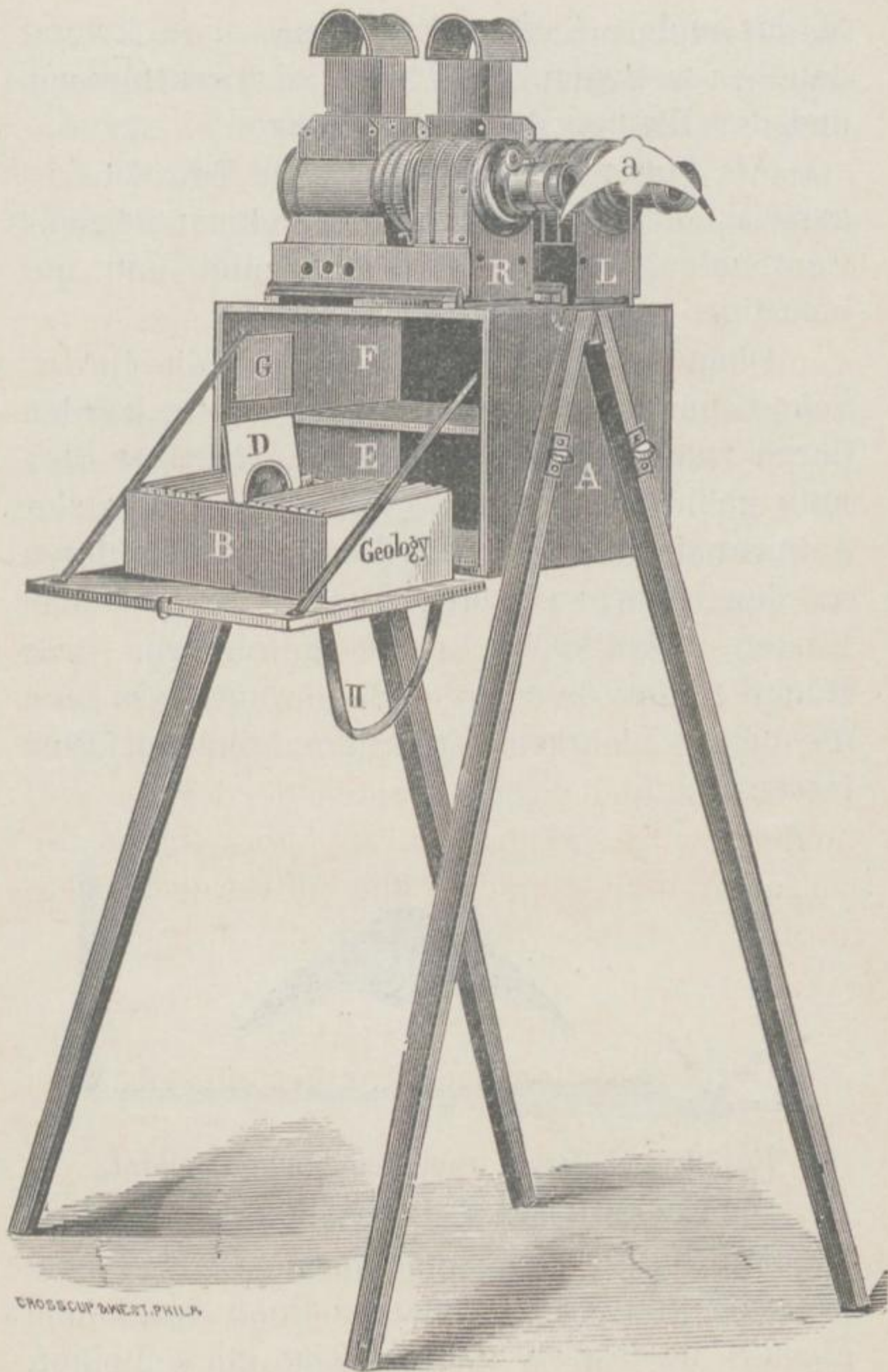
Fig. 19. Nebelbilder-Apparat.
