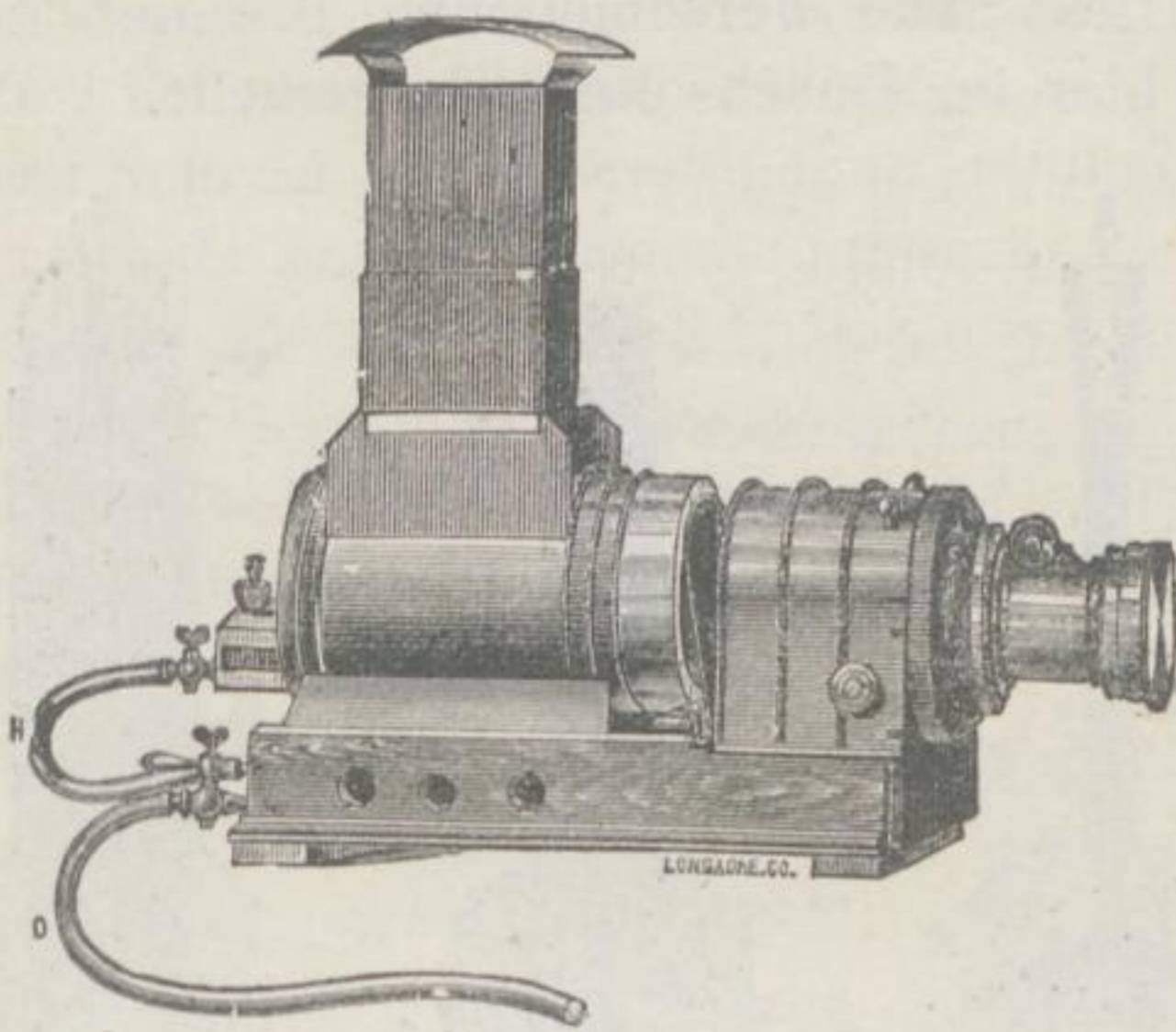
Fig. 43. Sciopticon mit Kalklicht.
